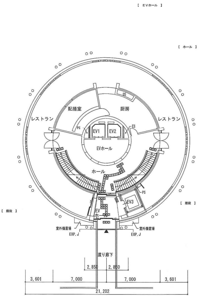
下層2階平面図
