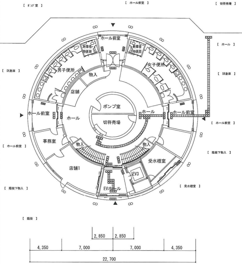
下層1階平面図
