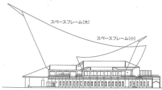
■東立面図
